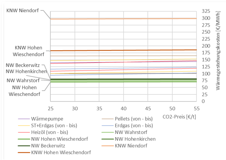
Abb. 69: Sensitivität CO 2 -Preis
