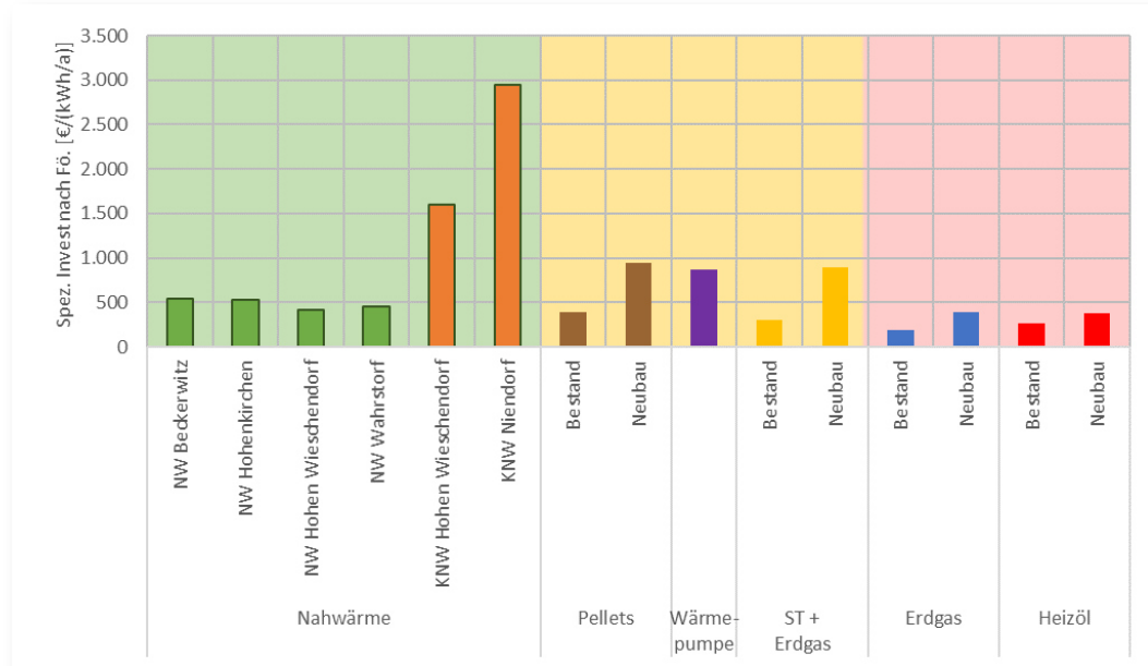
Abb. 63: Variantenvergleich spezifische Investitionskosten
