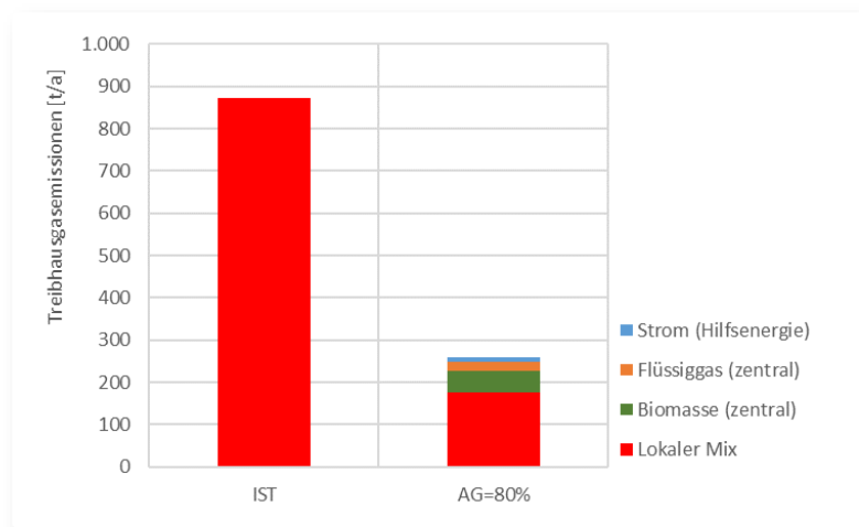
Abb. 38: Treibhausgaseinsparung Nahwärme Hohenkirchen (Anschlussgrad 80%)
