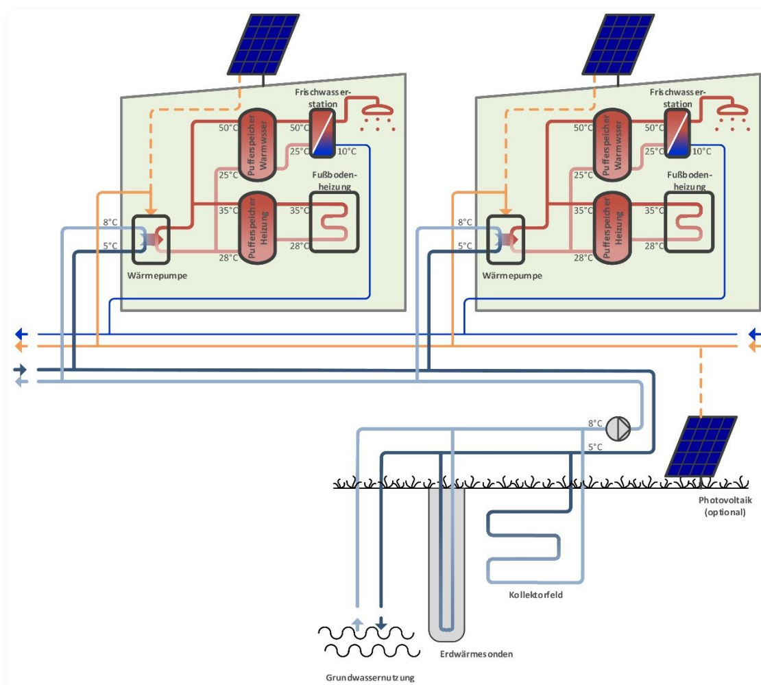
Abb. 51: Übersicht funktionale Konzeption kalte Nahwärme
