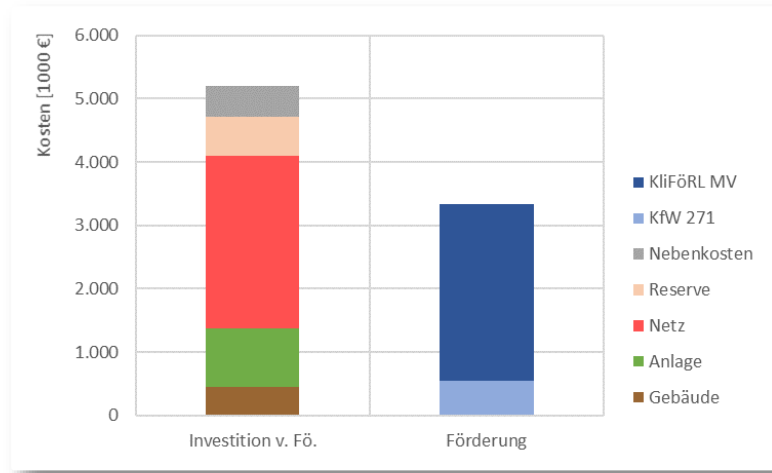
Abb. 34: Investitionsschätzung und Förderung Nahwärme Beckerwitz (Anschlussgrad 80%)
