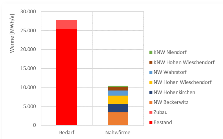
Abb. 60: Versorgungsumfang netzgebundener Anlagen
