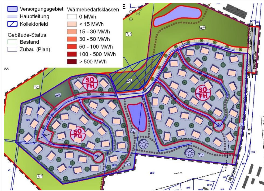
Abb. 56: Karte Versorgungsgebiet kalte Nahwärme Niendorf
