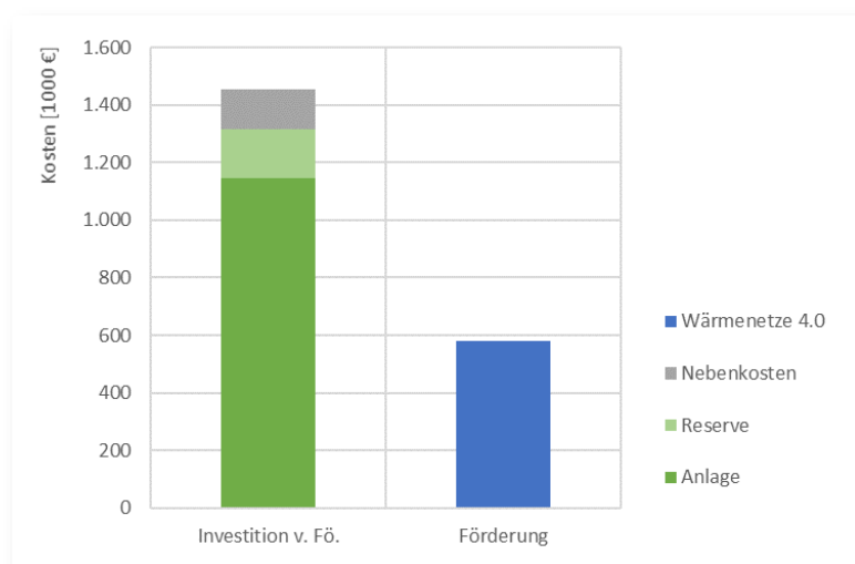
Abb. 58: Investitionsschätzung und Förderung kalte Nahwärme Niendorf
