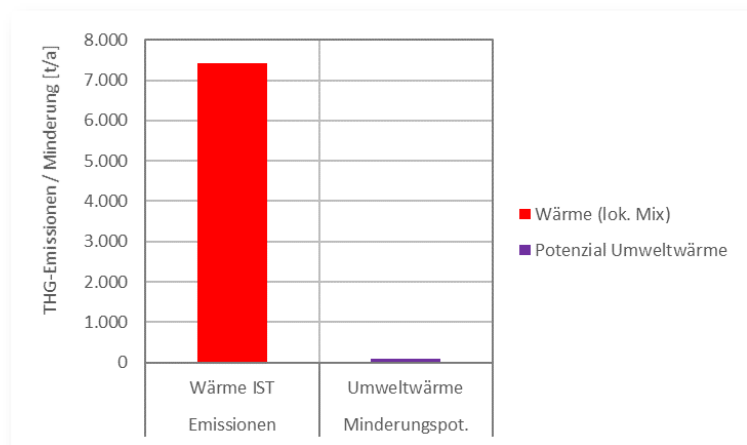
Abb. 18: Treibhausgasminderungspotenzial Umweltwärmenutzung
