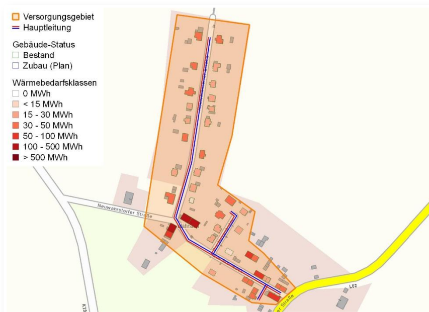
Abb. 46: Karte Versorgungsgebiet Nahwärme Wahrstorf
