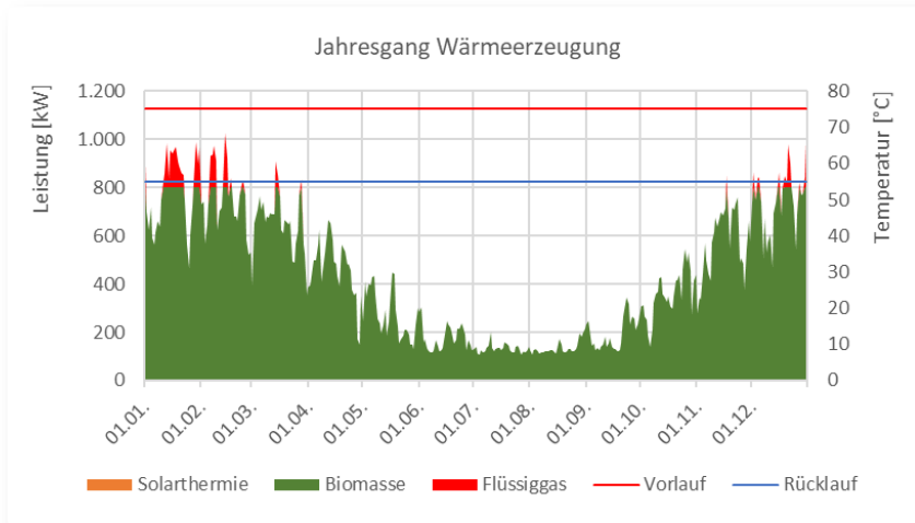
Abb. 32: Jahresgang Nahwärmeversorgung Beckerwitz (Anschlussgrad 80%)
