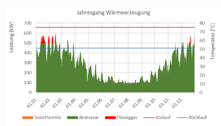
Abb. 42: Jahresgang Nahwärmeversorgung Hohen Wieschendorf (Anschlussgrad 80%)
