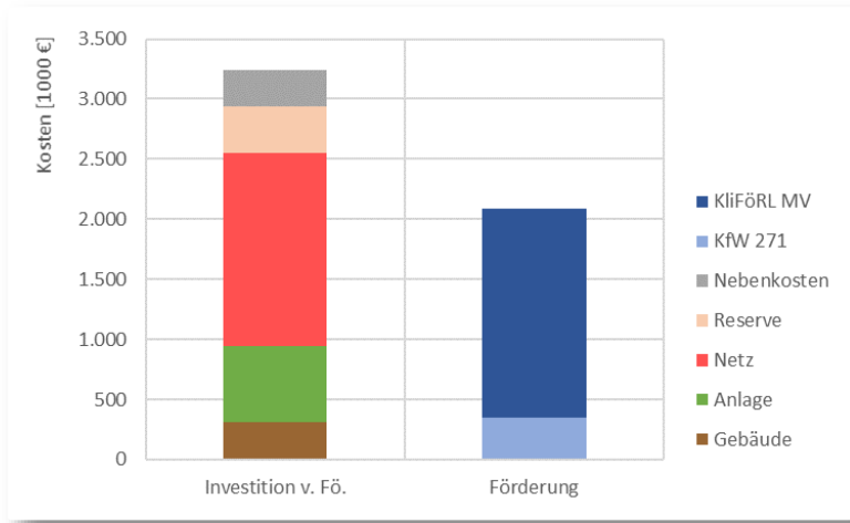
Abb. 39: Investitionsschätzung und Förderung Nahwärme Hohenkirchen (Anschlussgrad 80%)
