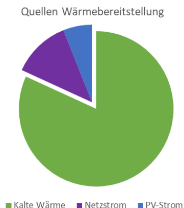
Abb. 57: Anteile Energieträger kalte Nahwärme Niendorf
