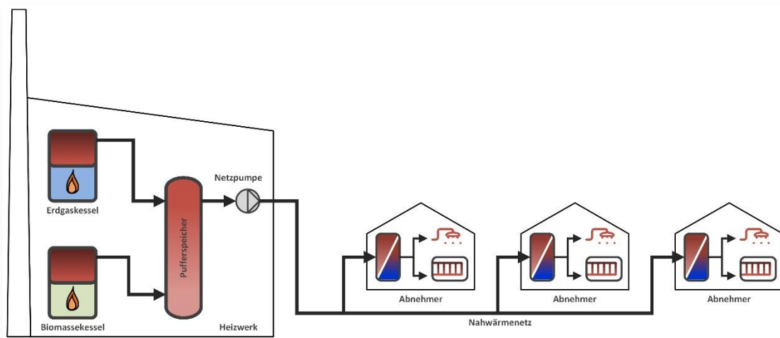
Abb. 23: Übersicht funktionale Konzeption Nahwärme
