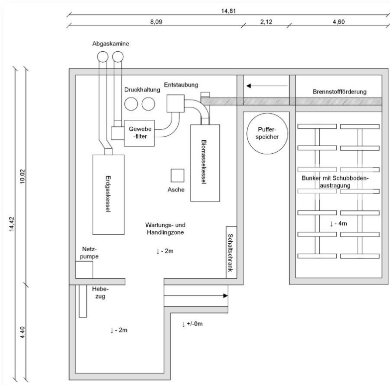
Abb. 25: Raumkonzept Heizzentrale
