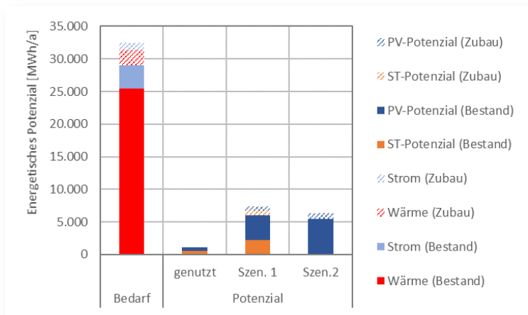
Abb. 15: Energetisches Potenzial solarer Aufdachanlagen
