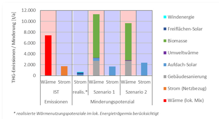
Abb. 22: Zusammenfassung Treibhausgas-minderungspotenzial
