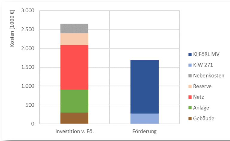
Abb. 44: Investitionsschätzung und Förderung Nahwärme Hohen Wieschendorf (Anschlussgrad 80%)
