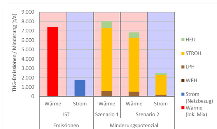
Abb. 14: Treibhausgasminderungspotenzial Biomasse
