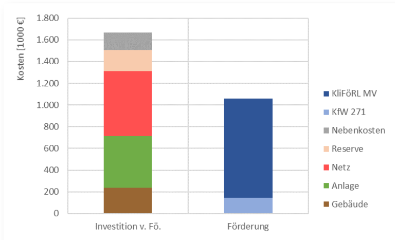
Abb. 49: Investitionsschätzung und Förderung Nahwärme Wahrstorf (Anschlussgrad 80%)
