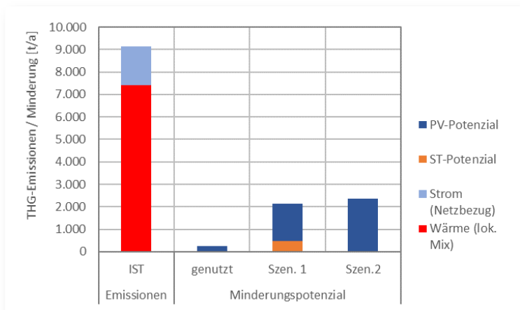
Abb. 16: Treibhausgasminderungspotenzial solarer Aufdachanlagen
