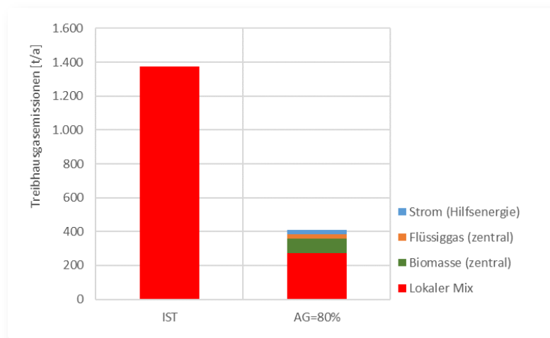
Abb. 33: Treibhausgaseinsparung Nahwärme Beckerwitz (Anschlussgrad 80%)
