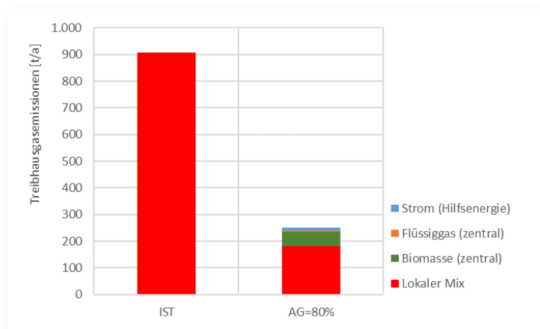
Abb. 43: Treibhausgaseinsparung Nahwärme Hohen Wieschendorf (Anschlussgrad 80%)
