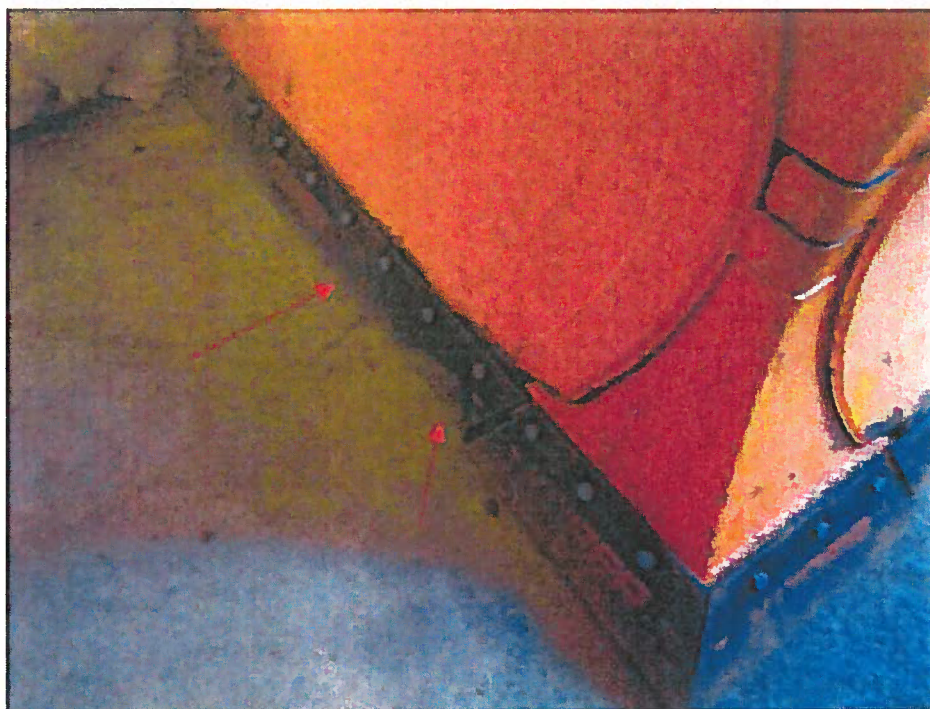
Bild 5 : Scharflügel rechts im unteren doppelwandigen,verstärkten Bereich und Schürfleiste gestaucht und stark verzogen
