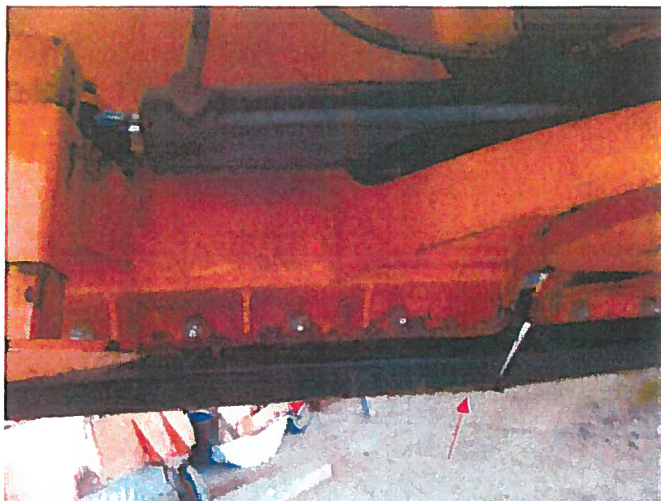
Bild 9 : Schadenbereich von hinten Scharfügel links im unteren,doppelwandigen,verstärkten Bereich verzogen
