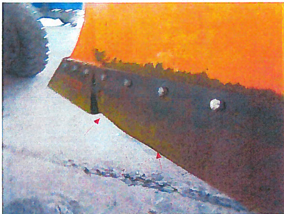
Bild 7 : Scharflügel links im unteren,doppelwandigen verstärkten Bereich und Schürfleiste gestaucht und stark verzogen
