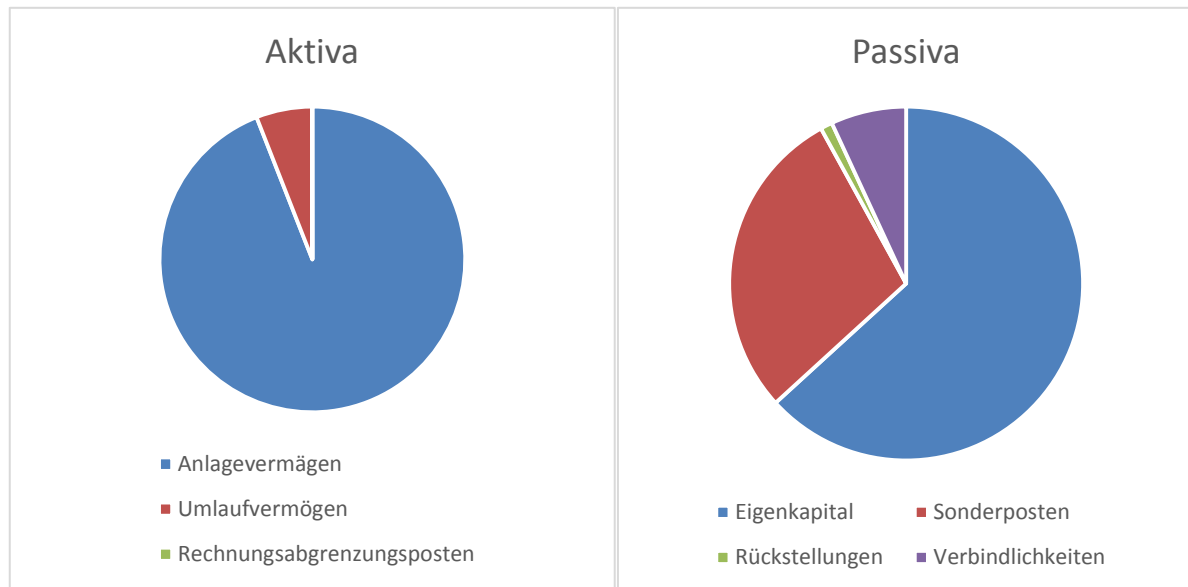
Bilanzstruktur
