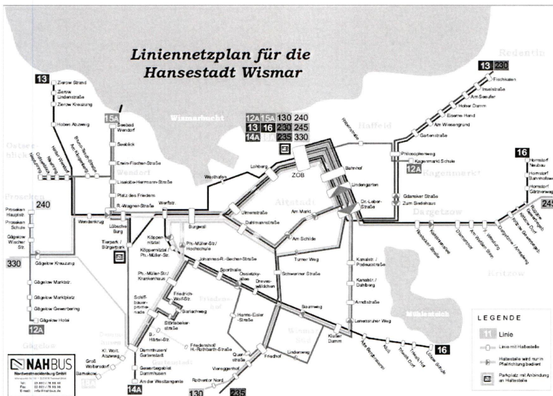
Abb.: erweiterter konzeptioneller Liniennetzplan
